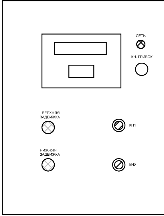
расположение элементов на передней панели шкафа
