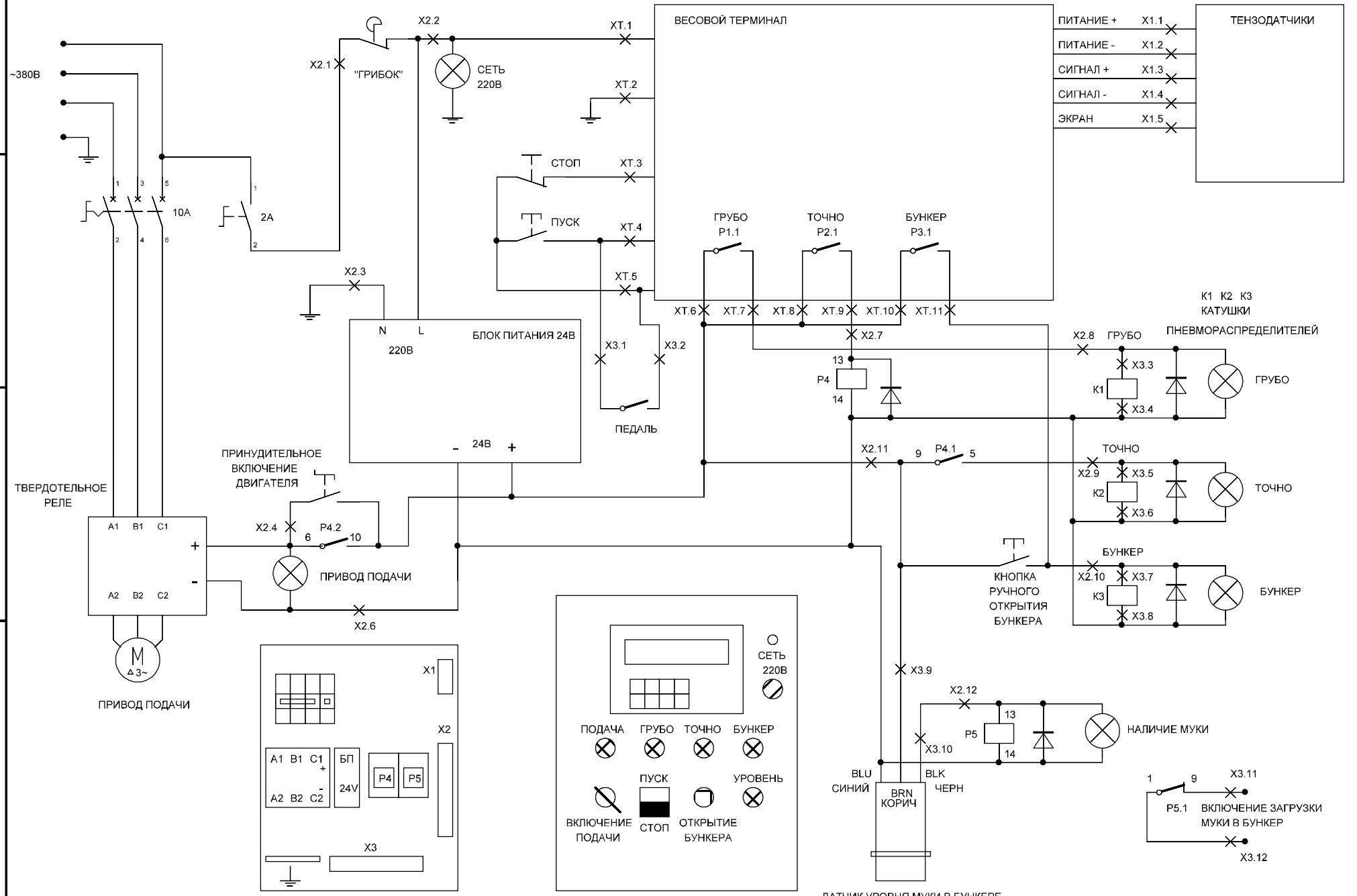
СХЕМА ЭЛЕКТРИЧЕСКАЯ ДОЗАТОРА 1-5 КГ
