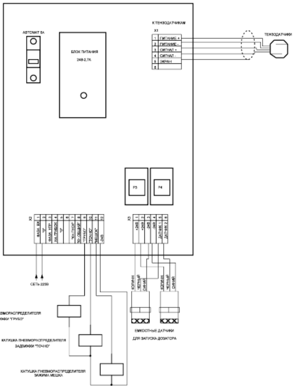
СХЕМА ПОДКЛЮЧЕНИЯ ШКАФА ДОЗАТОРА
