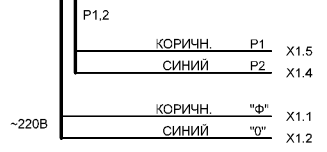
СХЕМА ПОДКЛЮЧЕНИЯ ВЕСОВОГО ТЕРМИНАЛА В ШКАФУ УПРАВЛЕНИЯ ДОЗАТОРОМ
