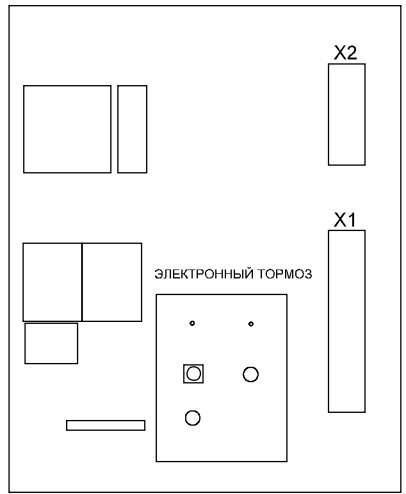
ВАРИАНТЫ РАСПОЛОЖЕНИЯ ЭЛЕМЕНТОВ ШКАФА
