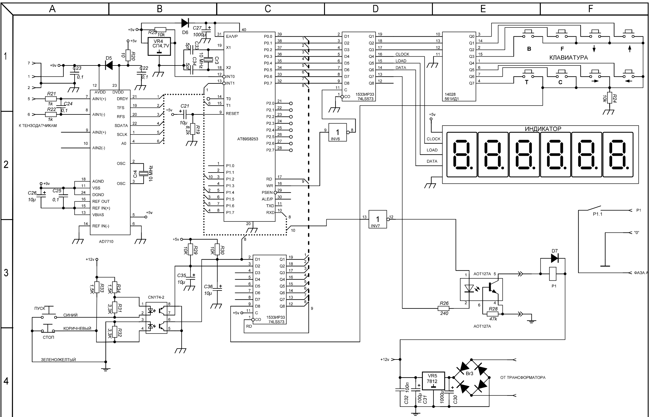
СХЕМА ТЕРМИНАЛА ДОЗАТОРА(ДОЗА-АГРО)
